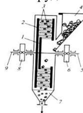
Рис. 3 Дисковая дробилка
