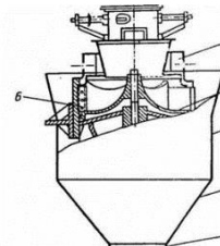
Рис. 6 Рамная центробежная свеклорезка
