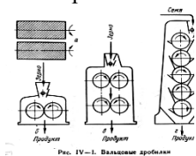
Рис.1 Вальцовые дробилки
