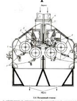
Рис. 2 Вальцовый станок
