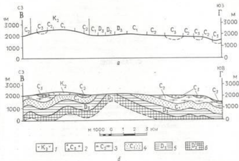
Геологический разрез
