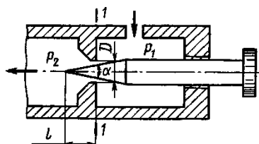
Рис. 2 Расчетная схема.
