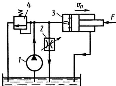
Рис. 3. Расчетная схема.
