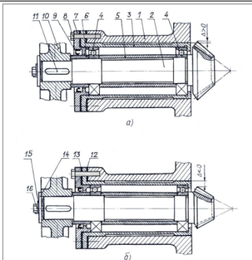
Рис. П.3.1. а) – без монтажного фланца. б) – с монтажным фланцем. Д. 1 – корпус; 2 – вал шестерни; 3 – стержень; 4 – подшипник радиально-упорный (2 шт.) 3-5 – втулка дистанционная; 6 – втулка упорная; 7 – фланец; 8 – болт М8х35 (4 шт.); 9 – манжета уплотнительная; 10 – колесо зубчатое; 11 – шпонка; 12 – прокладка; 13 – набор прокладок; 14 – шайба торцевая; 15 – шайба стопорная (отгибная); 16 – болт М8х25
