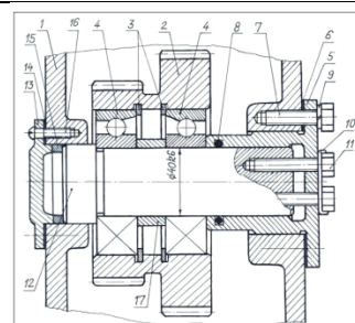
Рис. П.3.3. Ось блока шестерен 1 – корпус; 2 – блок шестерен; 3 – кольцо пружинное (2 шт.); 4 – подшипник радиально-упорный 1508 (2 шт.); 5 – фланец; 6 – прокладка; 7 – болт М10х40 (4 шт.); 8 – кольцо уплотнительное; 9 – шайба упорная (4 шт.); 10 – шайба стопорная (отгибная); 11 – болт М8х30; 12 – ось; 13 – вал; 14 – крышка; 15 – кольцо дистанционное; 16 – винт М8х30 (4 шт.); 17 – втулка дистанционная
