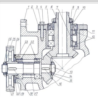
Рис. П.3.5. Конический редуктор 1 – корпус; 2 – стержень; 3 – болт М8х40 (4 шт.); 4 – шайба упорная; 5 – втулка ребристая; 6 – вал шестерни; 7 – втулка дистанционная; 8 – гайка шпоночная; 9 – шайба коническая; 10 – втулка коническая; 11 – прокладка; 12 – подшипник конический (2 шт.); 13 – вал ведомый; 14 – гайка шпоночная; 15 – шайба коническая; 16 – шпонка; 17 – втулка дистанционная; 18 – шпонка; 19 – манжета; 20 – прокладка; 21 – кольцо зубчатое; 22 – подшипник шариковый (2 шт.); 23 – винт М8х25 (4 шт.); 24 – крышка скользящая; 25 – шайба коническая; 26 – гайка шпоночная
