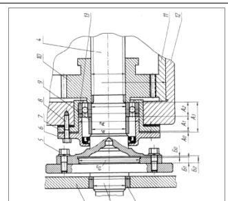
Узел 1. Привод с внутренним зубчатым механизмом. Вращение от вала 3, установленного в корпусе 2, через подшипник скольжения 1, передается шпоночному валу 4 посредством шестерен 5. Зубчатое колесо 10 передается на шпоночный вал 6 и входит в зацепление с внутренним зубчатым колесом 11, от которого вращение на счет посадок 1 передается на корпус 12 привода. Радиальный подшипник колена 13 посажен в корпус 12 на скользящей посадке 4. Фланец 14 в корпусе 12 соединен с коленом 15 уплотнением с кольцом 16. Дистанционное кольцо 9 устанавливается на валу 4 свободно на скользящей посадке.
