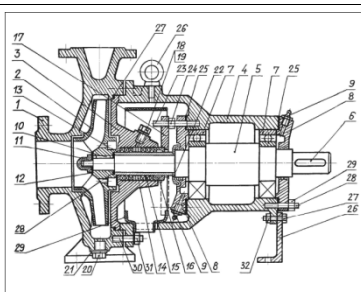
Рис. П.3.7. Насос консольный центробежный марки НК 1 – корпус насоса; 2 – колесо; 3 – корпус уплотнения; 4 – кронштейн; 5 – вал; 6 – шпонка; 7 – подшипник шариковый (2 шт.); 8 – крышка подшипника (2 шт.); 9 – пресс-масленка (2 шт.); 10 – шпонка; 11 – гайка коническая; 12 – прокладка; 13 – втулка скользящая; 14 – фланец уплотнения; 15 – кольцо сальниковое (6 шт.); 16 – втулка коническая; 17 – рукоятка; 18 – пробка М10; 19 – прокладка; 20 – пробка М16; 21 – прокладка; 22 – кольцо шпоночное; 23 – шпонка М10 (2 шт.); 24 – гайка М10 (2 шт.); 25 – прокладка (2 шт.); 26 – кронштейн; 27 – болт М8х30 (2 шт.); 28 – шпилька М10 (8 шт.); 29 – гайка М 10 (8 шт.); 30 – шпилька М12 (6 шт.); 31 – гайка М12 (6 шт.); 32 – гайка М8 (2 шт.)
