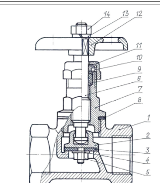
Рис. П.3.6. Вентиль в сборе 1 – корпус; 2 – клапан; 3 – прокладка клапана; 4 – шайба; 5 – гайка М6; 6 – золотник; 7 – крышка; 8 – прокладка; 9 – уплотнение сальниковое; 10 – втулка коническая; 22 – гвоздики; 12 – рукоятка; 13 – шайба упорная; 14 – гайка М 10
