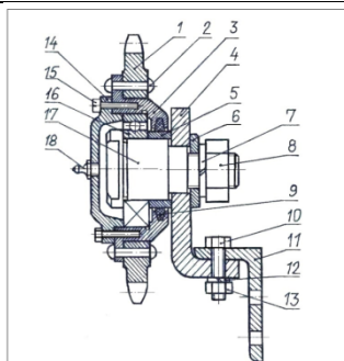
Рис. П.3.2. Выходная в сборе 1 – манжета; 2 – манжета (6 шт.); 3 – стержень; 4 – кронштейн; 5 – втулка; 6 – шайба; 7 – шайба упорная; 8 – гайка М10; 9 – уплотнение кольцевое; 10 – болт М8х35 (2 шт.); 11 – упорная пружинная (40х6); 12 – шайба упорная (4 шт.); 13 – гайка М8 (2 шт.); 14 – крышка глухая; 14 – крышка; 15 – винт М8х30 (6 шт.); 16 – подшипник шариковый радиальный № 205; 17 – ось; 18 – пресс-масленка
