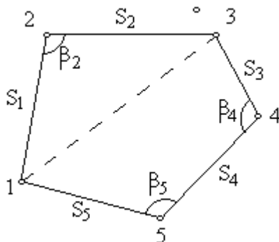
Рис. 14 Схема для определения общей площади полигона
