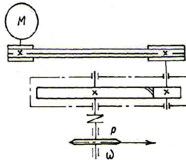
6. Привод зернопогрузчика.
