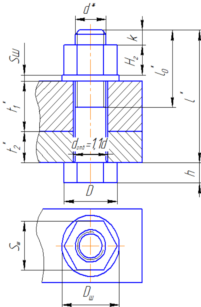
Рис.1 – Размеры болтового соединения
