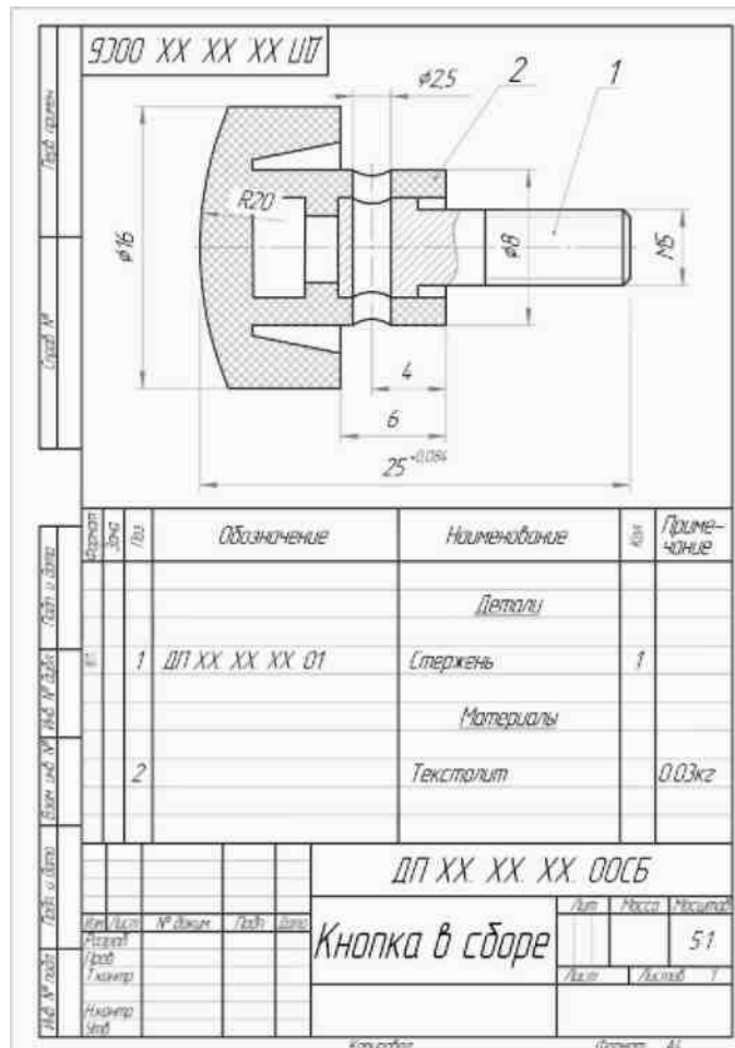
Рис. 4. Спецификация сборочной единицы
