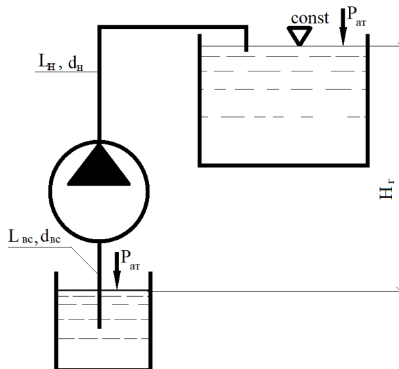
Рис. 1. Расчетная схема.
